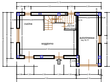
PIANTA PIANO TERRENO
