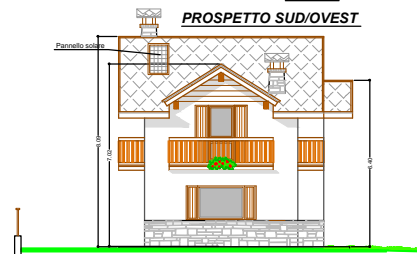
PROSPETTO SUD/OVEST
