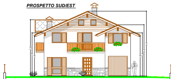
PROSPETTO SUD/EST
