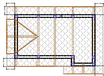
PIANTA COPERTURA
